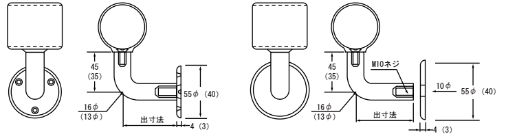
■ステンレス丸パイプ受 L軸 木ネジ座
