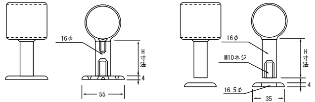
■ステンレス丸パイプ受 直軸 木ネジ座
