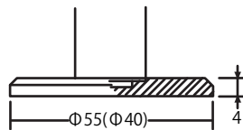
■固定アンカー座
